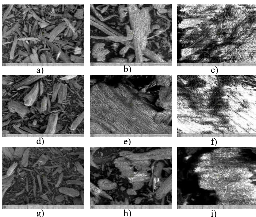
Fig. 1. Imagini SEM ale biomasei lemnoase mărunțite la diferite mărimi: (a) caise - 100 X; (b) caise - 500 X; (c) caise - 2000 X; (d) piersic - 100 X; (e) piersic - 500 X; (f) piersic - 2000 X; (g) prune - 100 X; (h) prune - 500 X; (i) plus - 2000 X. Sursă: [7]
