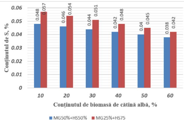
Fig. 4. Conținutul de sulf în brichetele produse din amestecuri de MG +HS cu adaus de reziduuri de cătină albă în diferite proporții
