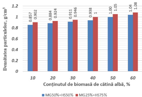
Fig. 3. Densitatea particulelor brichetelor din amestecuri de MG +HS cu adaus de reziduuri de cătină albă în diferite proporții
