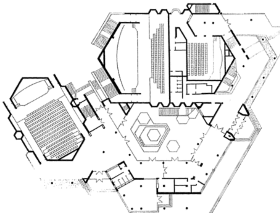
Fig. 4. Planul cinematografului ”Tiraspol” cu trei săli (100, 300 și 600 spectatori), arh.V.Sumîșevskii.
